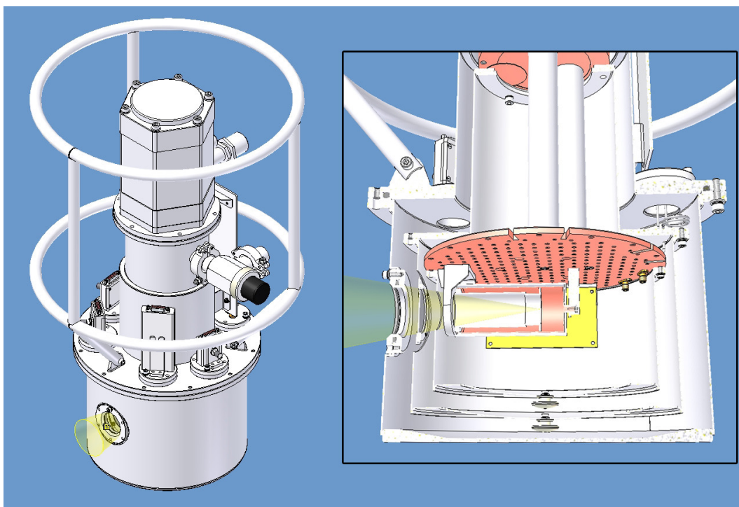
Рисунок 4 – Эскиз криостата для системы замкнутого цикла.
